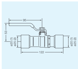
0659.10 - Llave de paso esférica para sistema de termofusión para caños de 20 y 25 mm de diámetro.
