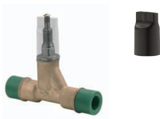
0489.02FVBASE - Llave de paso para sistema de termofusión para caños de 20 y 25 mm de diámetro. Sin volante y campana (*)
