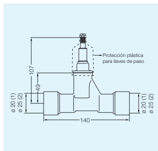
0489.02FVBASE - Llave de paso para sistema de termofusión para caños de 20 y 25 mm de diámetro. Sin volante y campana (*)
