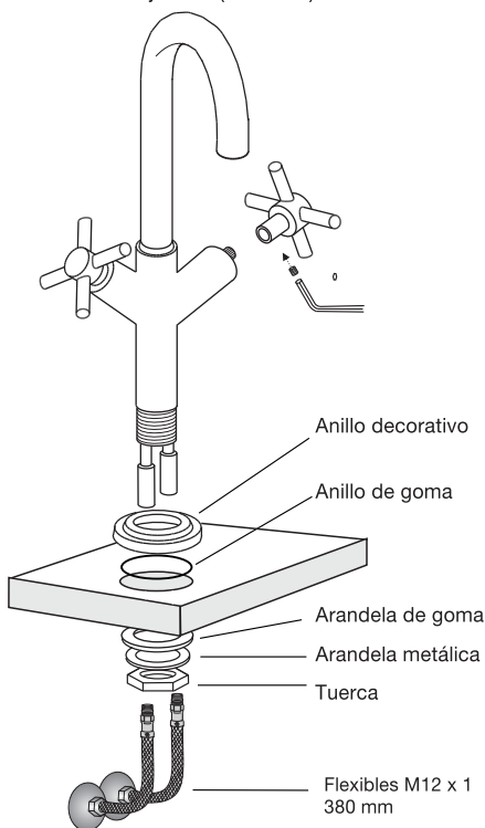
Detalle de fijación (0446.02)
